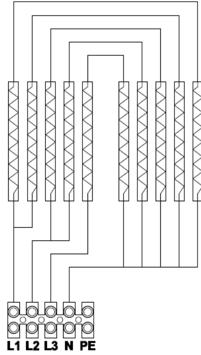
5 takım Rezistans
