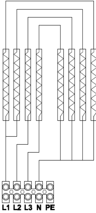
4 takım Rezistans
