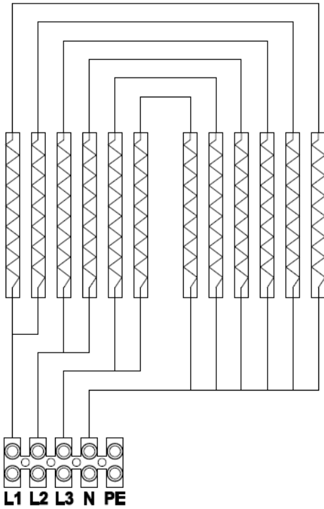
6 takım Rezistans
